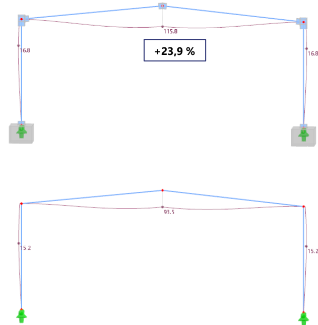
Verformungen
