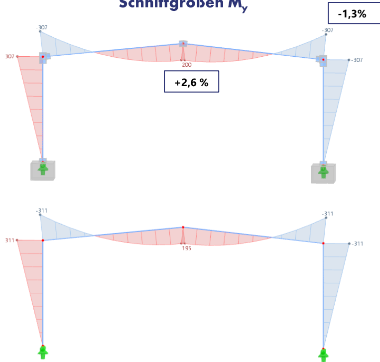
Schnittgrößen M_y
